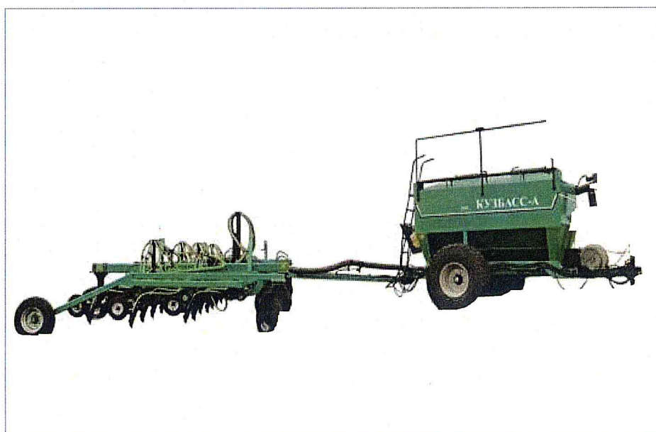
Рисунок 1 – Посевной комплекс «Кузбасс» ПК-9,7 (общий вид).
