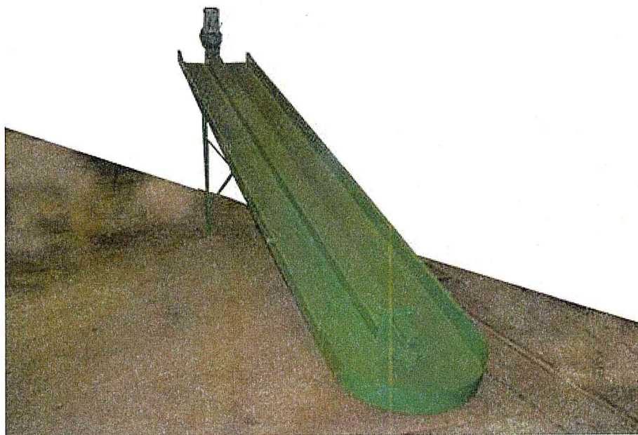
Рисунок 1. Транспортер наклонный ТСН-160 (без цепи).
