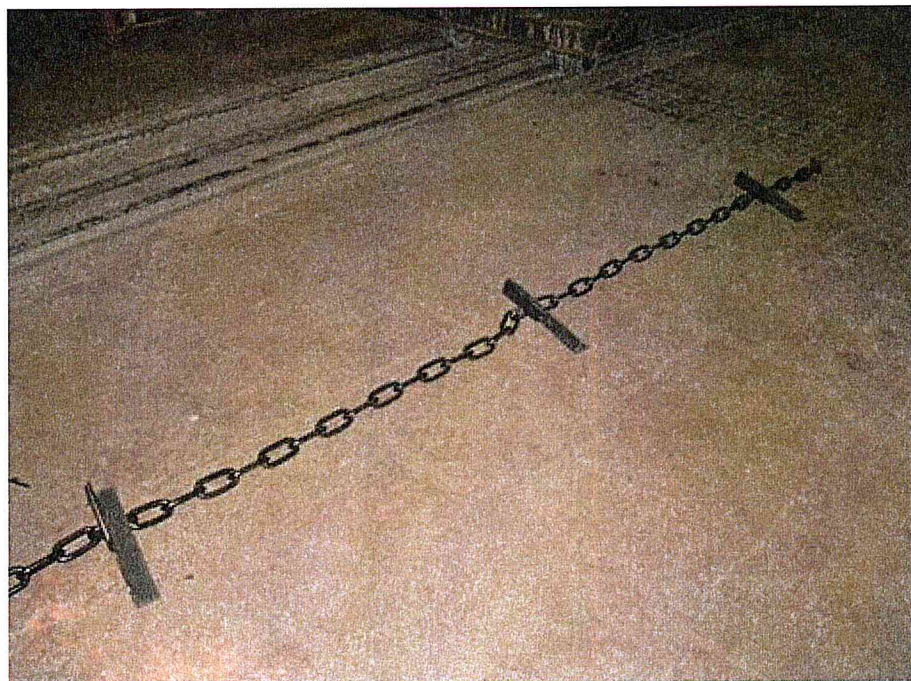
Рисунок 3. Цепь со скребками транспортера горизонтального ТСН-160.
